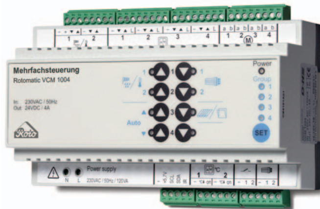
Mehrfachsteuerung Rotomatic VCM 1004 zur bauseitigen Montage im Schaltschrank
