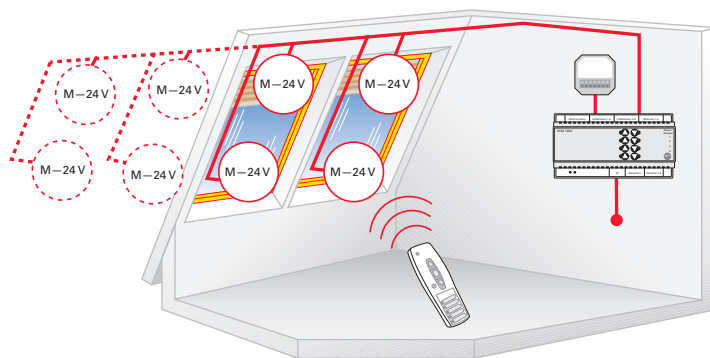
Bis zu 8 Antriebe lassen sich mit einer VCM 1004 ansteuern. Zum Beispiel 4 Fenster mit Kettenantrieb MA 25 N und jeweils einer Jalousette Elektrisch und einem Falstore Elektrisch. Mit einem Handsender und einem Funkempfänger 4fach 24V kann die Bedienung komfortabel per Funk erfolgen.
